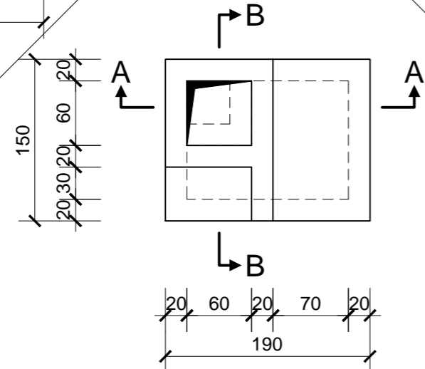
Felülnézet, M=1:50
