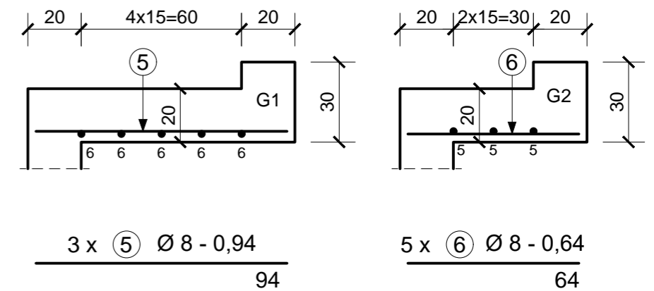
L2 lemez, M=1:20
