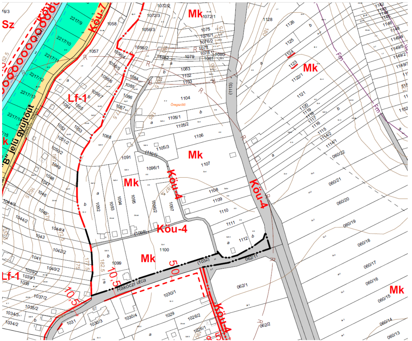
I. ábra: Szabályozási terv
