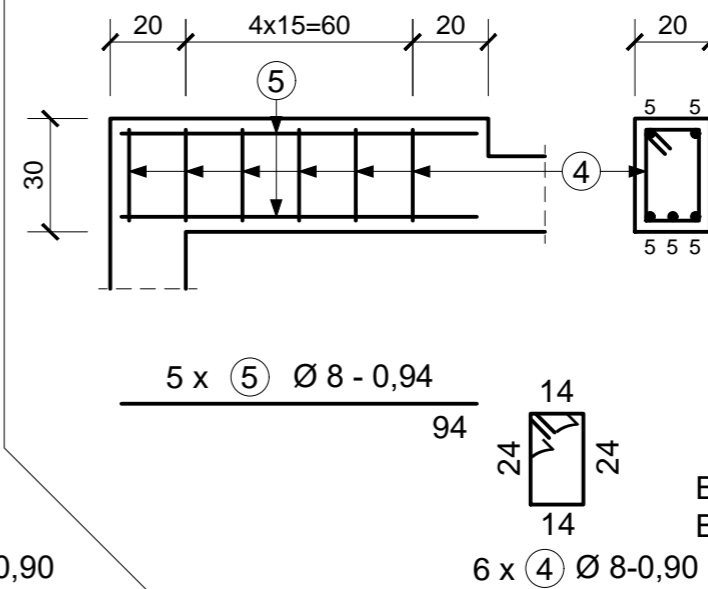
L1 lemez, M=1:20
