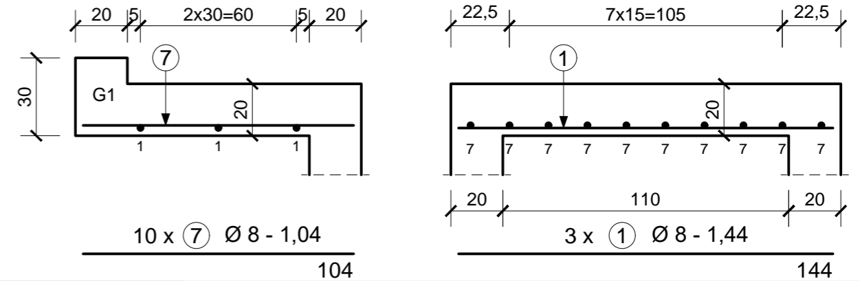
L2 lemez, M=1:20
