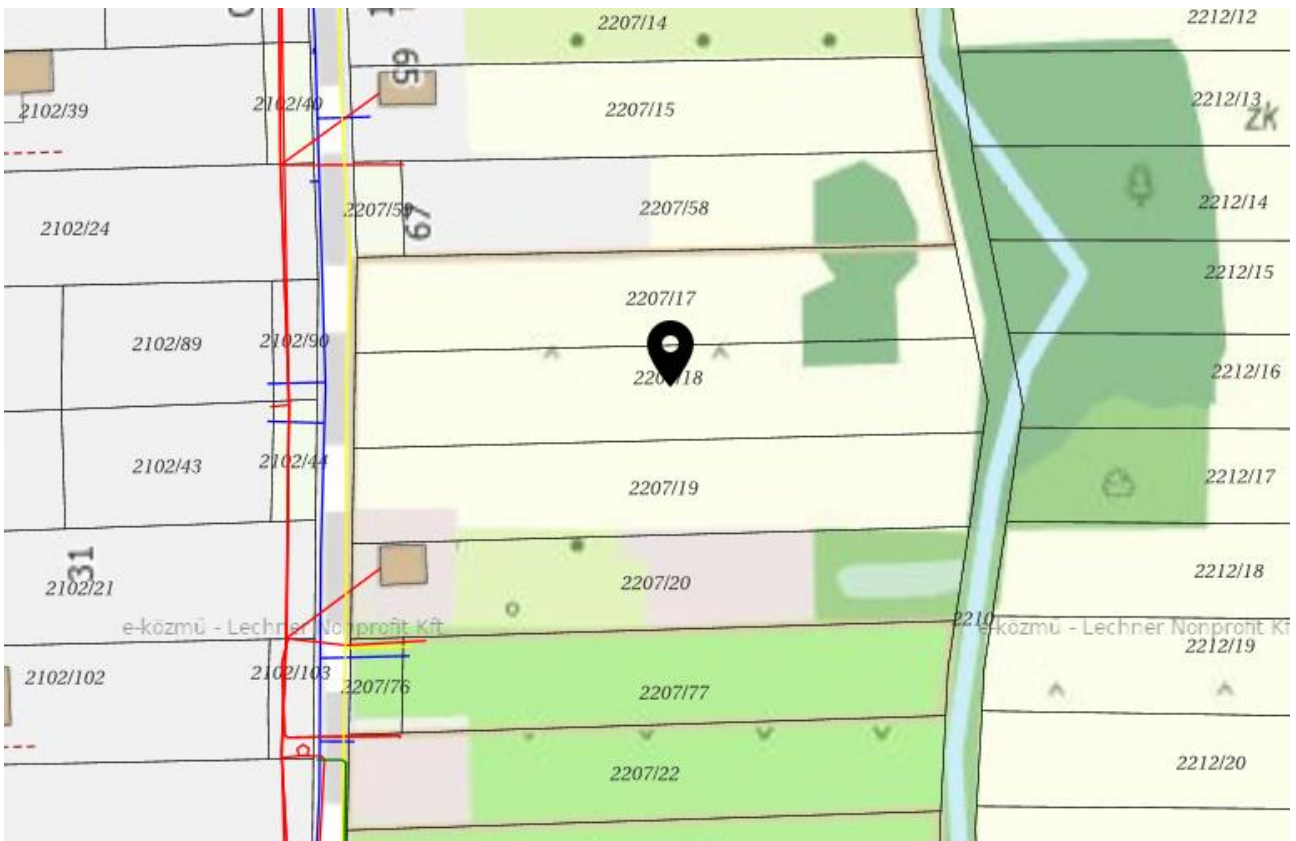
3. ábra: A 2207/18 hrsz előtt futó közművek; kék: ivóvíz; piros: áram; bordó: szennyvíz; sárga: gáz (forrás: e-kozmü)
