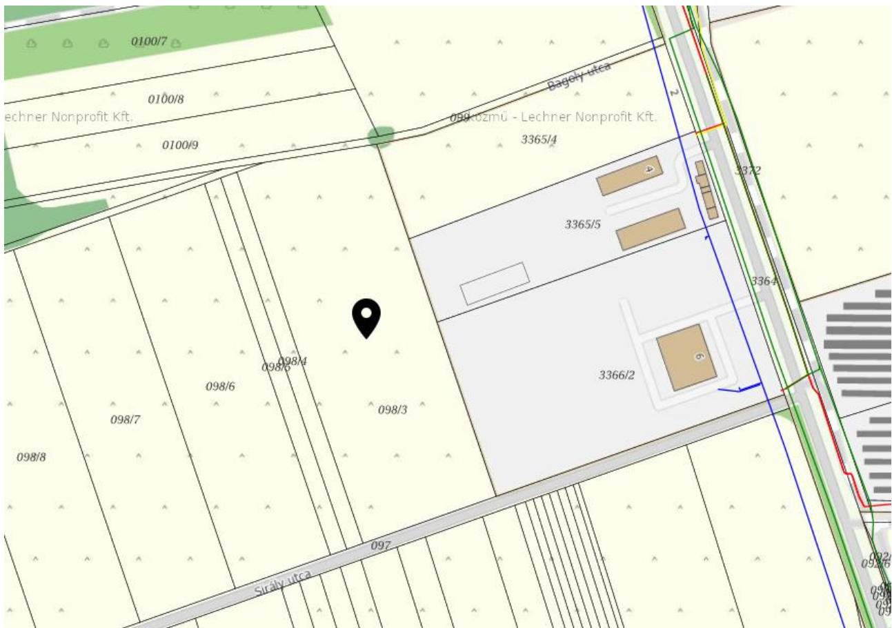
5. ábra: Az 098/3 hrsz előtt futó közművek; kék: ivóvíz; piros: áram; sárga: gáz (forrás: e-közmű)
