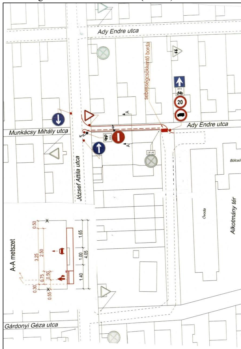
7. ábra: Az óvodai parkoló egyirányú megközelítéséhez szükséges úthálózat kialakítása
